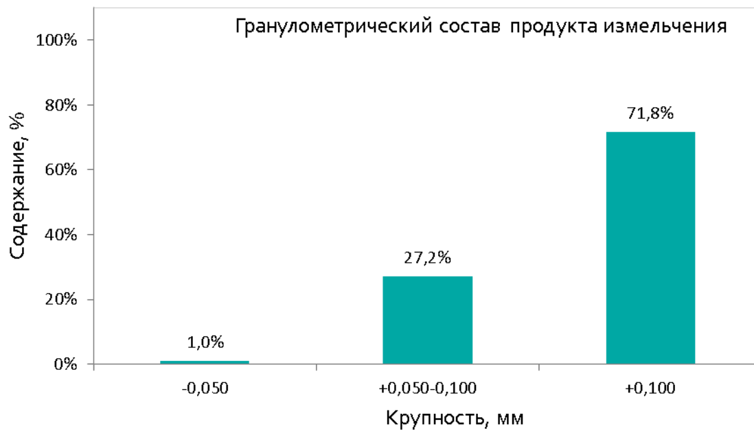
Рис. 4. Гранулометрический состав продукта измельчения
