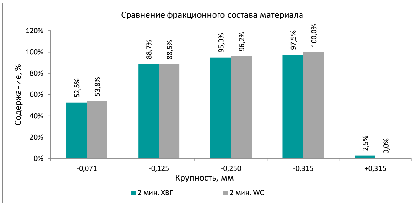
Рис. 7. Фракционный состав продукта измельчения
