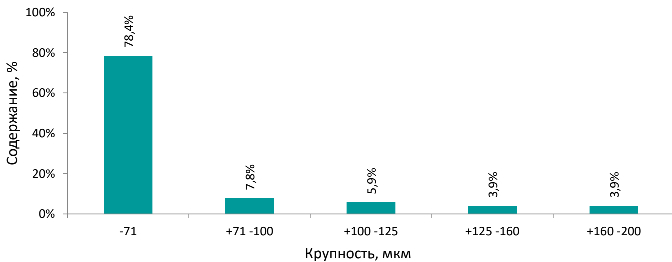
Рис. 5. Гранулометрический состав продукта измельчения
