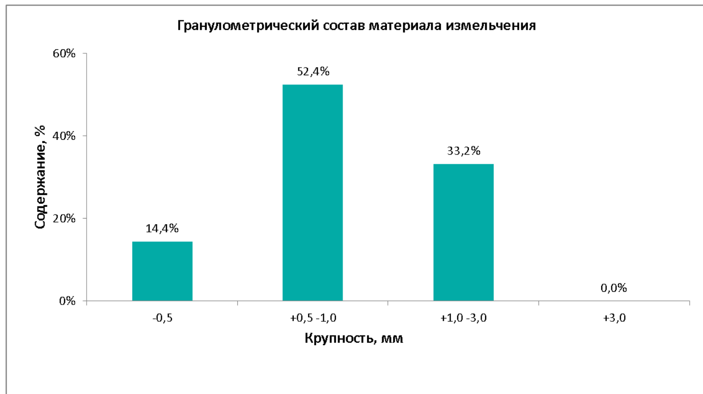
Рис. 4. Гранулометрический состав продукта измельчения
