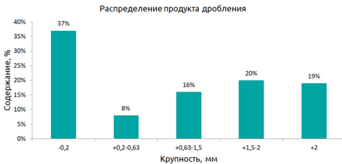
Рис. 6. Распределение продукта дробления
