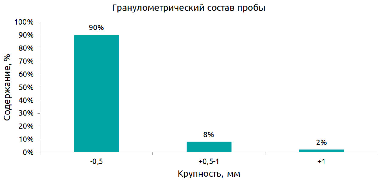
Рис. 3. Гранулометрический состав пробы
