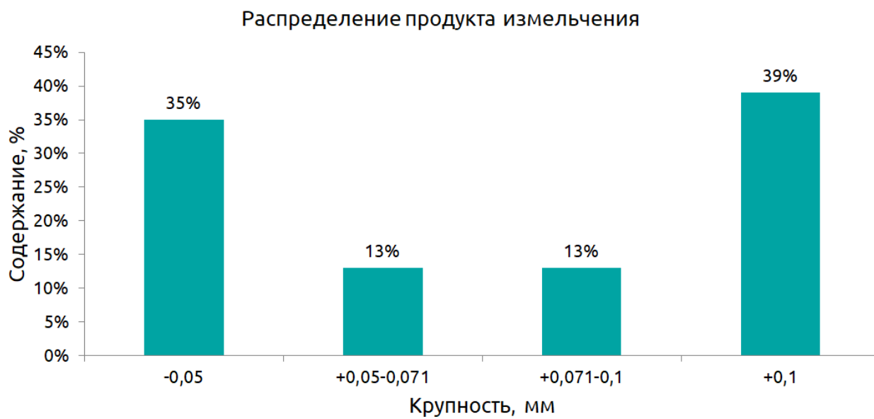
Рис. 6. Распределение продукта измельчения
