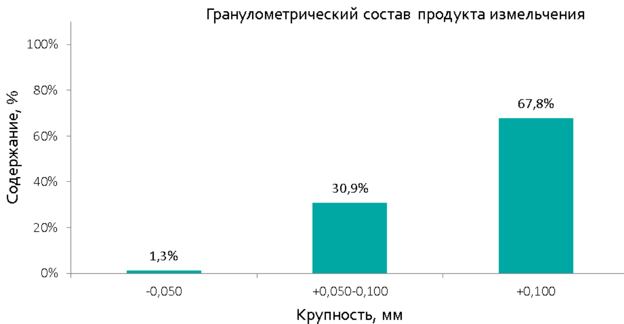
Рис. 7. Гранулометрический состав продукта измельчения
