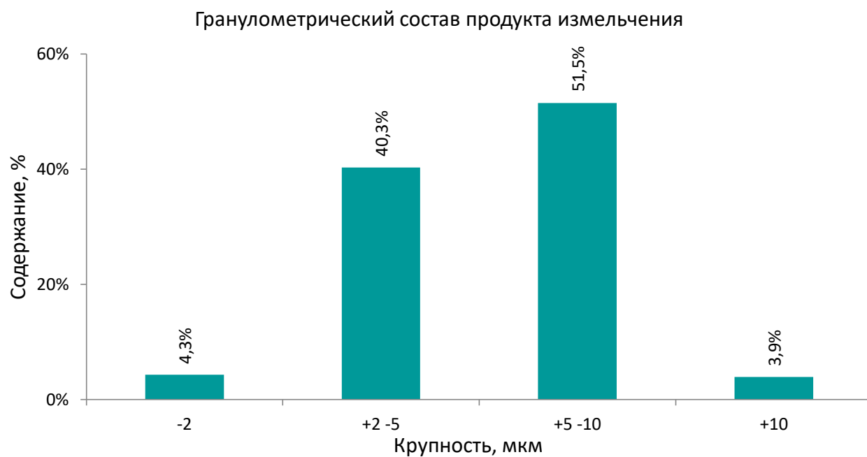
Рис. 5. Гранулометрический состав продукта измельчения
