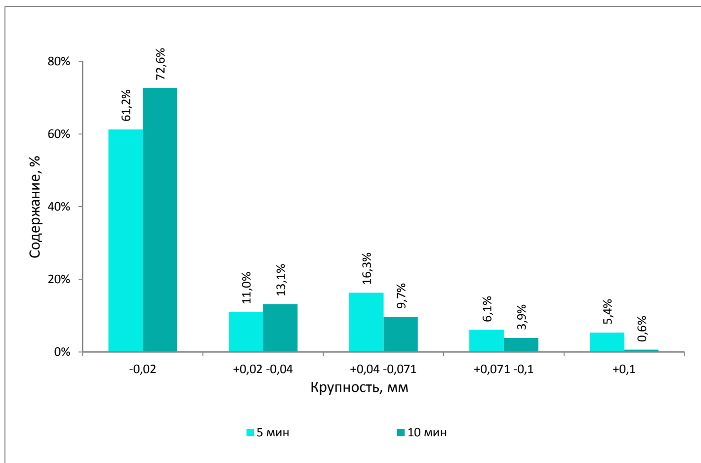
Рис. 3. Сравнение гранулометрического состава материала по разделу 2
