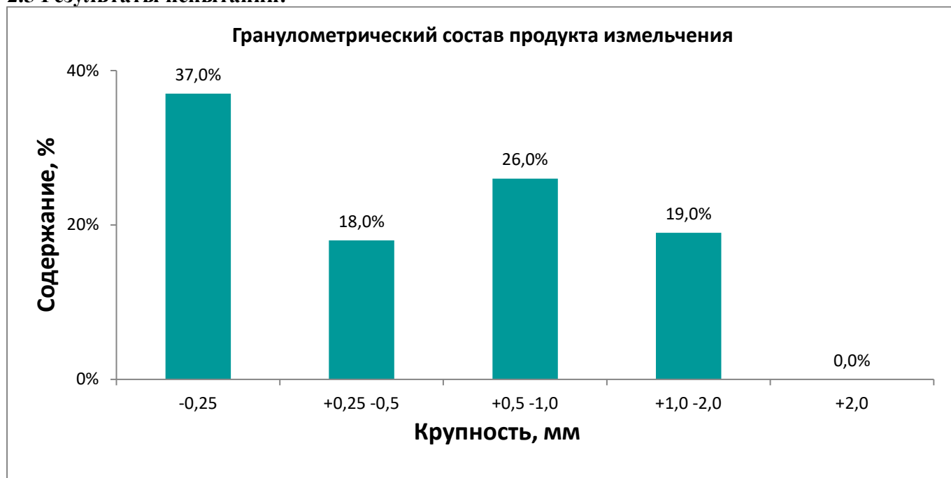
Рис. 5. Гранулометрический состав продукта измельчения
