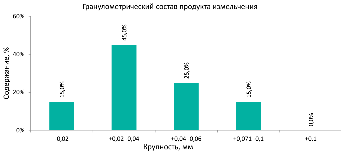
Рис. 4. Гранулометрического состав продукта измельчения
