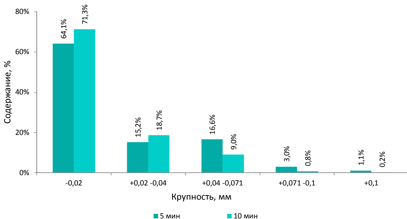
Рис. 3. Сравнение гранулометрического состава продукта измельчения по разделу 2
