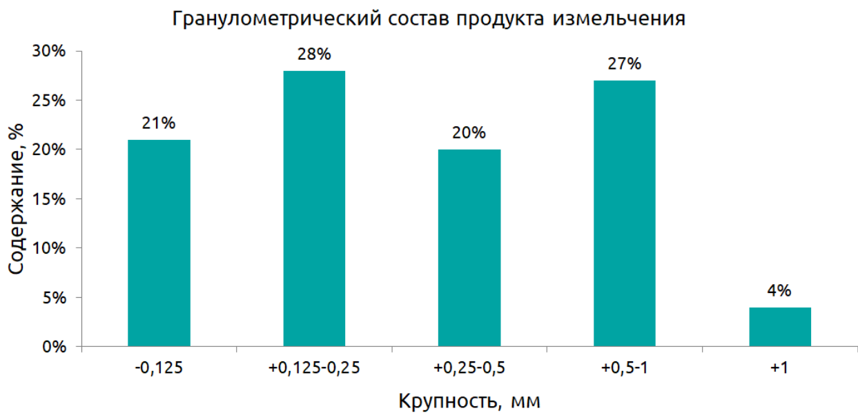
Рис. 5. Гранулометрический состав продукта измельчения
